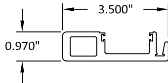
9A OPTIONAL SASH/ STILE INTERLOCK 6063-T5
