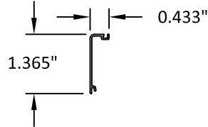
5 SASH END CAP 6063-T5
