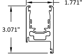
1A OPTIONAL SASH RAIL/STILE 6063-T5
