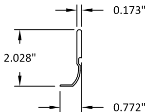
35 OPTIONAL RISER 6063-T5
