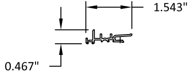
7 POCKET INTERLOCK 6063-T5
